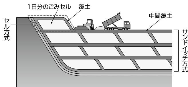
▲ 埋め立て工法 セル方式及びサンドイッチ方式
